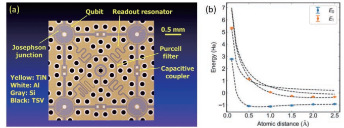
(a) 量子ビットチップのユニットセル構造。これを繰り返し敷き詰めることでより大きいチップを構成する。(b) SSVQE法により求めた、水素分子の基底状態と第一励起状態のエネルギー準位の原子間距離依存性。
