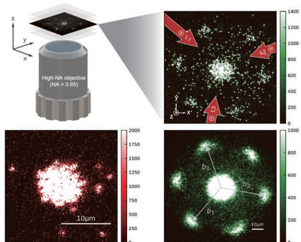
量子気体顕微鏡による測定。飛行時間測定法によるコヒーレンス測定 (右上) と光格子内での実空間測定 (左下) の両方を行うことができる。右下はコヒーレンス測定の実験結果を平均化したもの。
