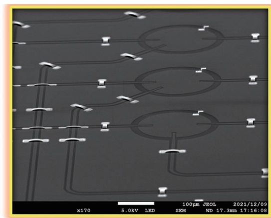
100ビットチップの部分拡大図。量子ビットをエアブリッジが見える。
