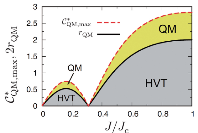
反強磁性相互作用強度と電流相関の関係。隠れた変数理論(HVT)で記述できる領域と、量子力学(QM)でしか記述できない領域を示す。
