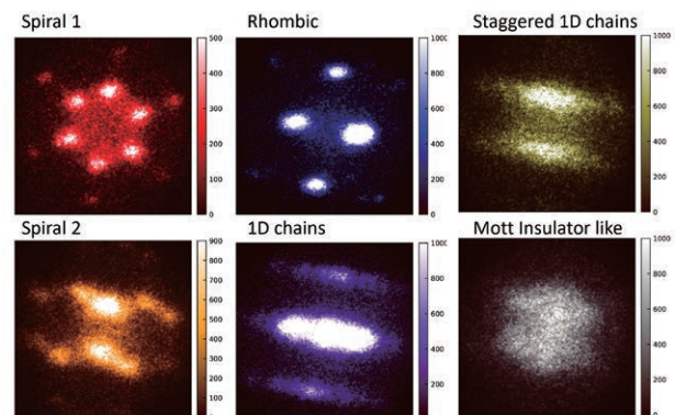
三角格子XYスピンモデルにおける様々な相に対応した干渉パターン
