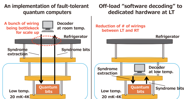
超伝導誤り耐性量子コンピュータの構成（左：従来、右：提案手法）
