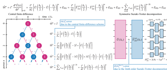
量子冪乗法の概念図
