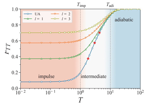
ハバード模型の基底状態フィデリティ(縦軸)の駆動時間(横軸)依存性。変分AGPによる駆動補助なしの場合(unassisted, UA)と駆動次数 l=1, 2, 3 の場合について結果を示している。
