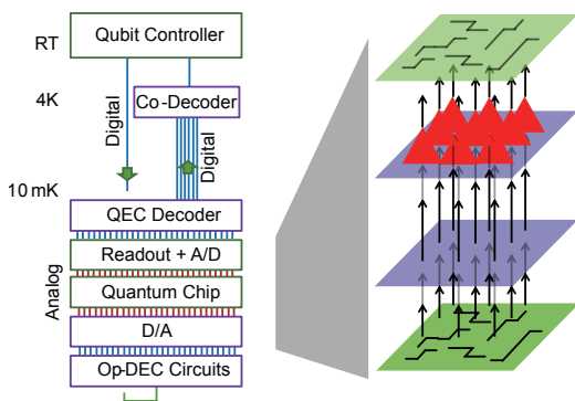
積層型モジュールシステム概念
